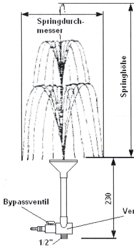
Abb. Düse II
